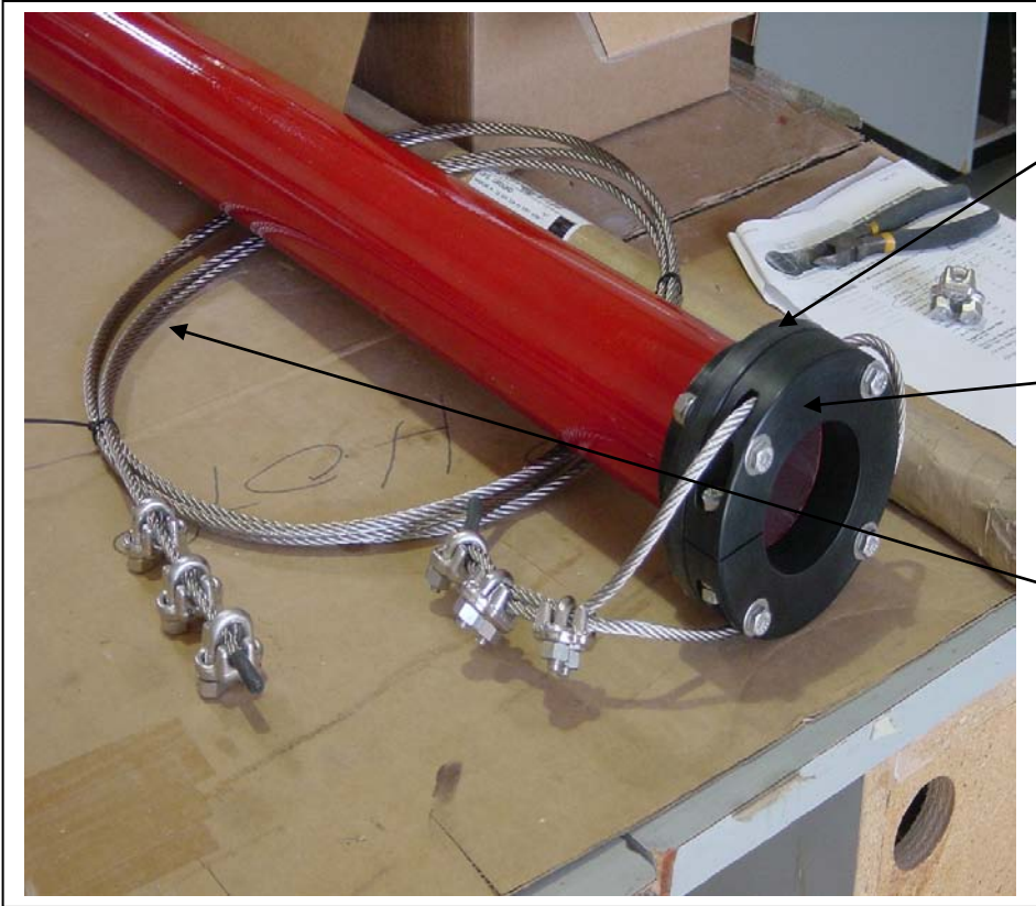
Profiler Flange
